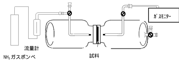
図1 動的消臭性評価装置の概要
