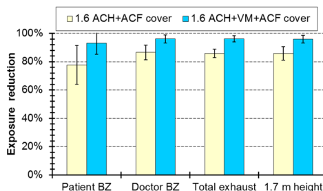
図 8 ACF-15 を掛布団カパー (ACF cover) または換気マットレスと掛布団カパーを組み合わせたとき (VM + ACF cover) のアンモニア減少率
