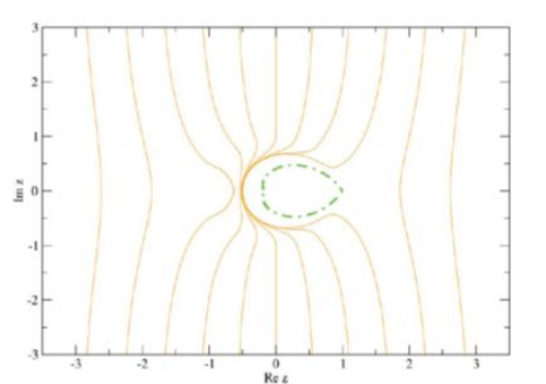
図1 2次元等方性媒質による透明マントを通るの光の経路
