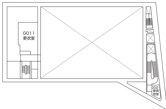
地下1階
